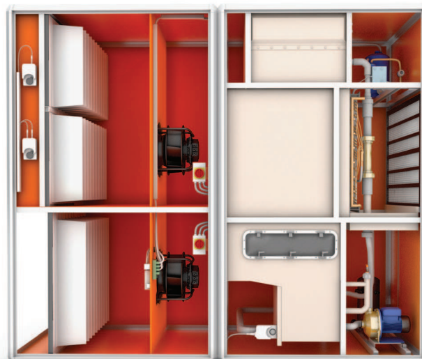
Adcoolair 75 13 01 – упрощенный вид
