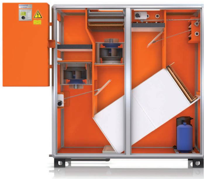
ThermoCond 29 20 01 – упрощенный вид
